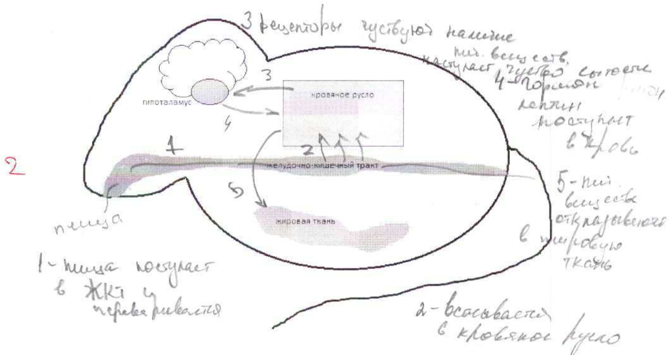
Рисунок. Схема регуляции чувства сытости у млекопитающих (2 балла).
